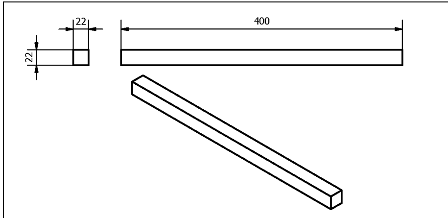
Tasseau (4) : 2 verts, 2 jaunes
