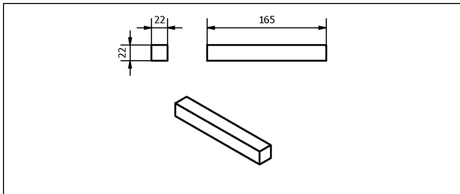
Tasseau (5) : 2 verts, 2 jaunes
