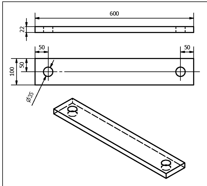
Estrade (7) : en un exemplaire
