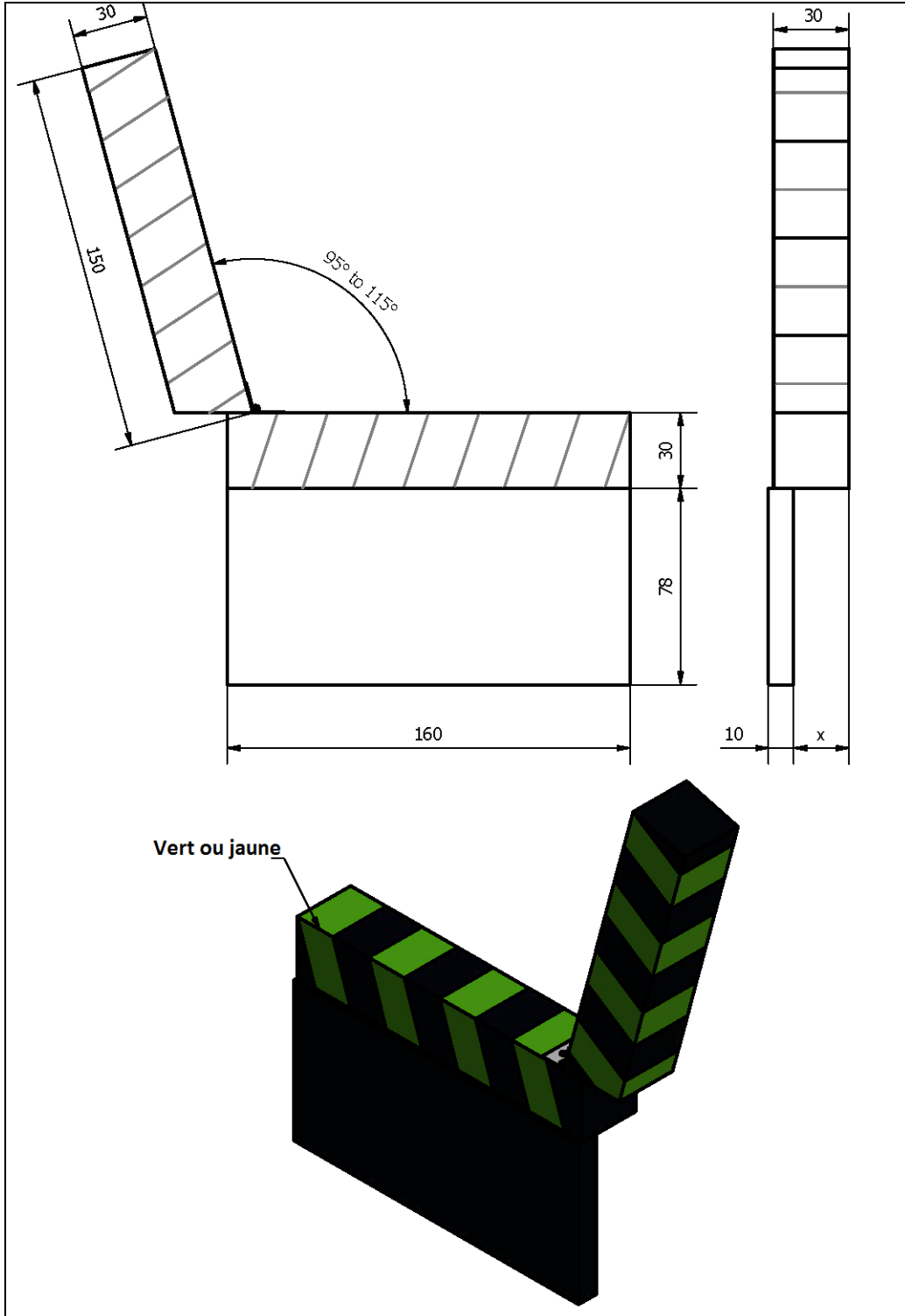
Les claps de droite (11) : 2 verts, 1 jaune
