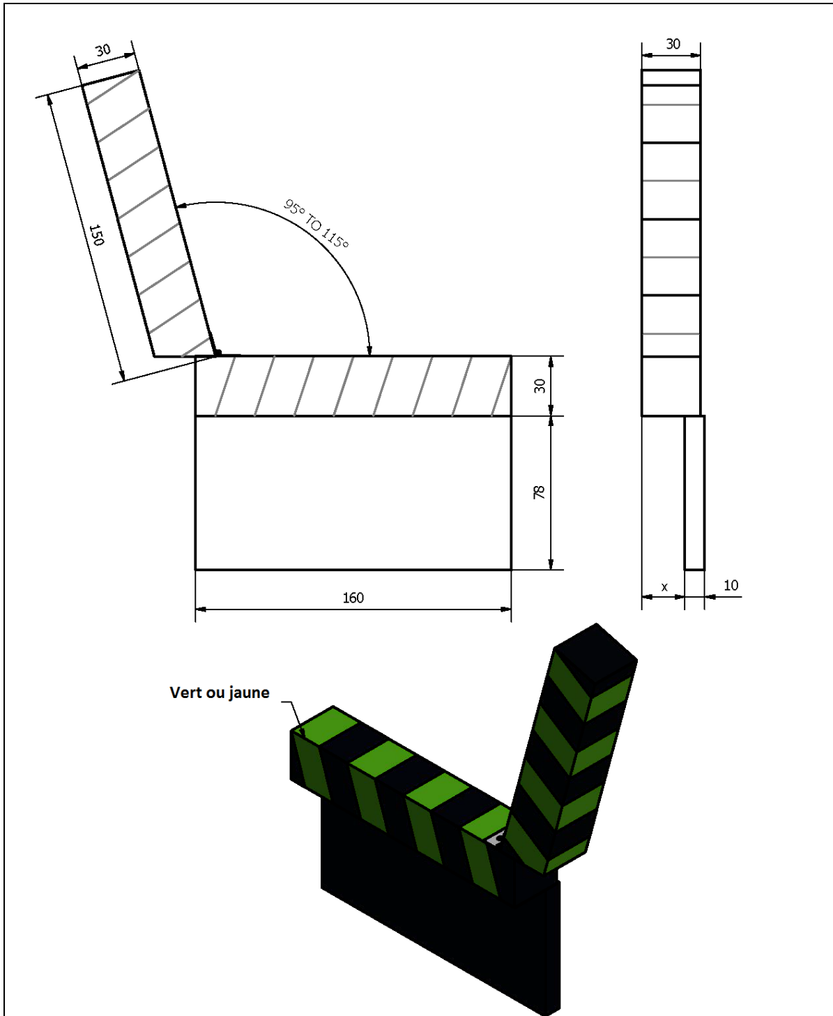
Les claps de gauche (10) : 1 vert, 2 jaunes
