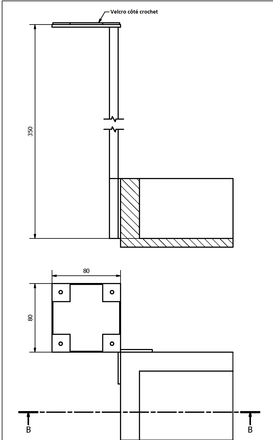
Balise de coin (2) : en quatre exemplaires
