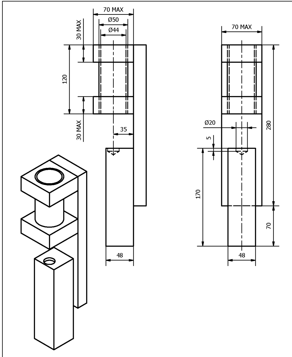
Les distributeurs de pop-corn (9) : en quatre exemplaires
