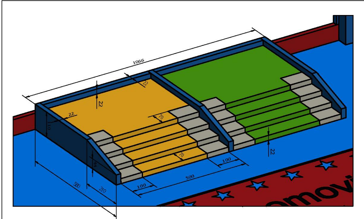
Marches (8) : en un exemplaire
