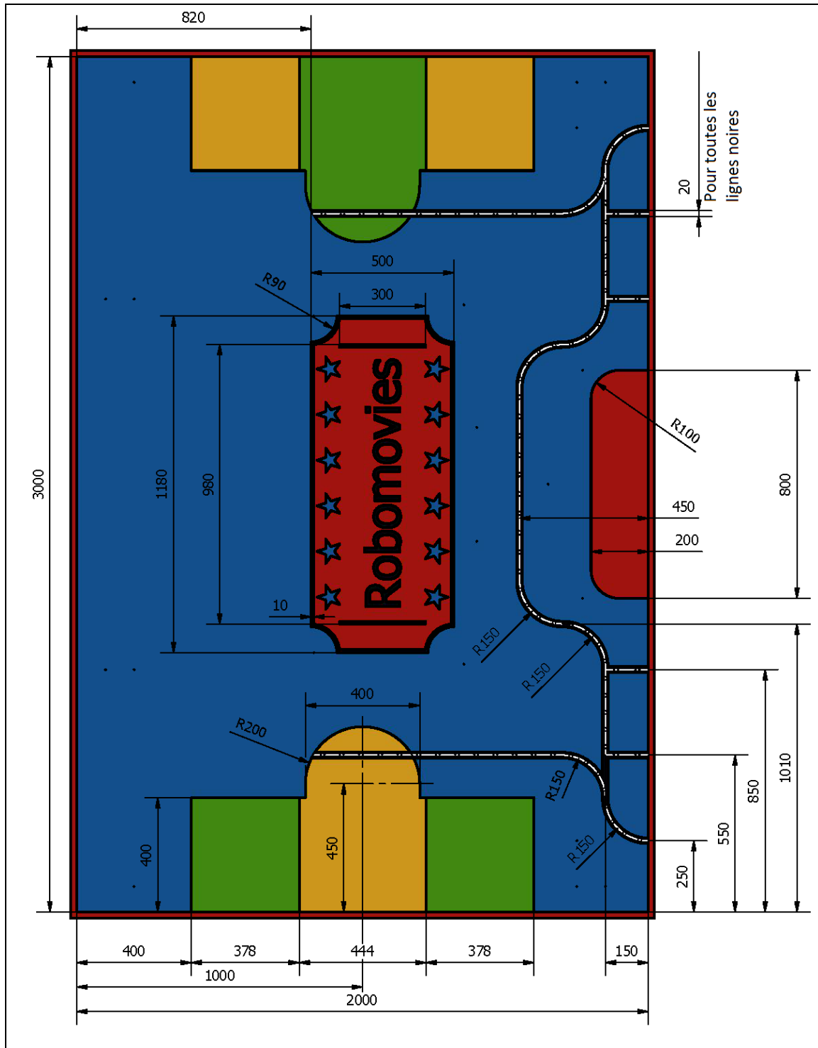
Aire de jeu (3)
