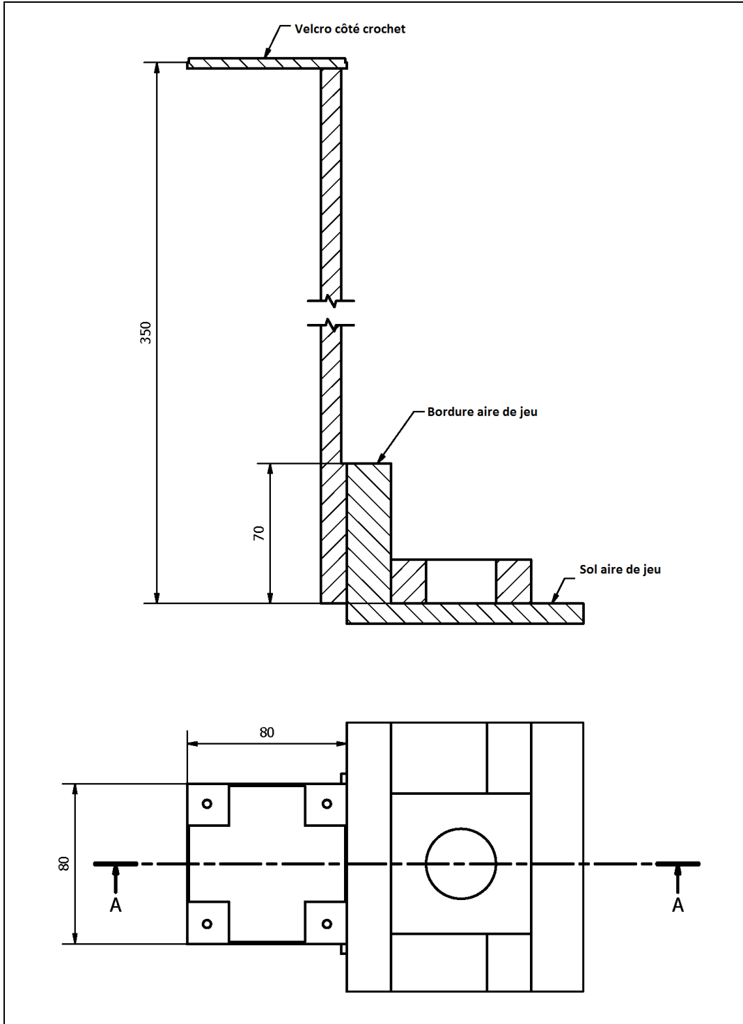
Balise du milieu (1) : en deux exemplaires
